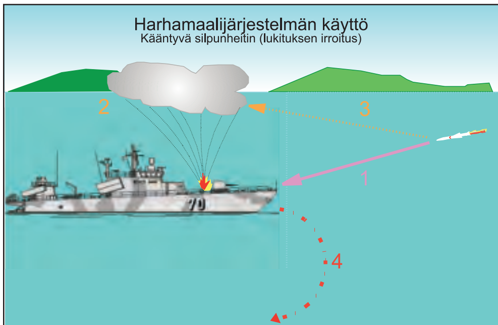
Esimerkki harhamaalijärjestelmän käytöstä (Rauma-lka).
