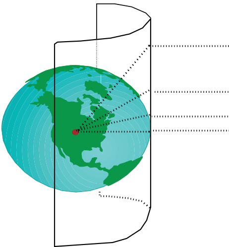
Mercatorin projektiio.
