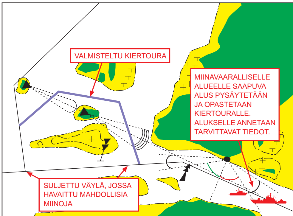
Opastaminen kiertouralla.
