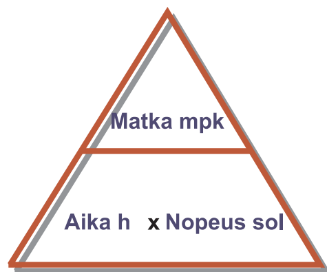
Nopeuskolmio.
