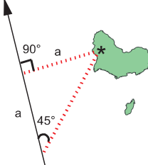
Kipparisuuntima
